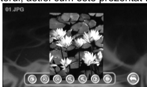
Figura 4-1 Vizualizator imagini
