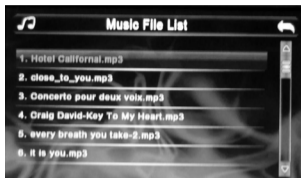
Figura 3-2 Directorul audio
